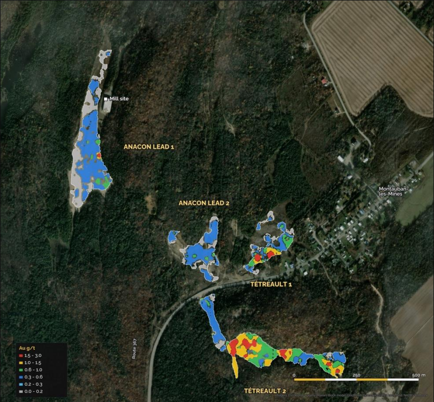
Photo : vue en plan du modèle de blocs, en couleurs selon la teneur en or (Au g/t)
